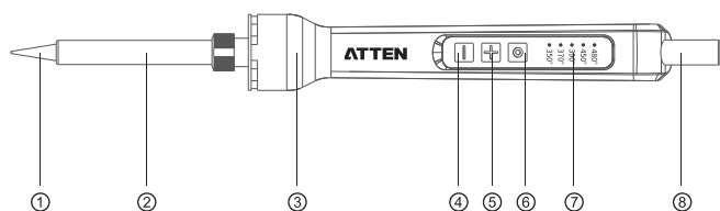
图1-1 (产品主视图)
